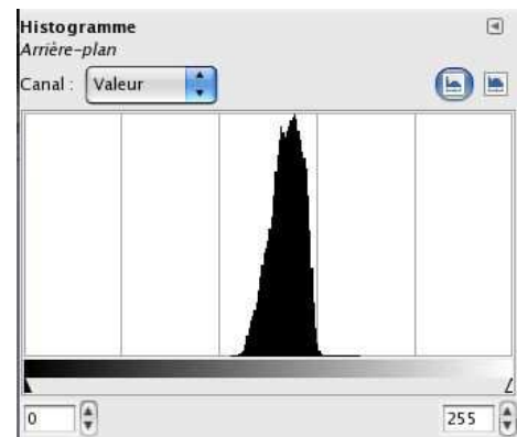
Histogramme D
